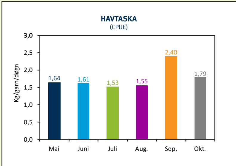
Mynd 4. Miðal veiða upp á roynd (CPUE) frá dagbókunum fyri havtasku pr. mánað í 2021. Litirnir sipa til, hvar ið gørnini hava staðið ávísa mánan í Mynd 5.
