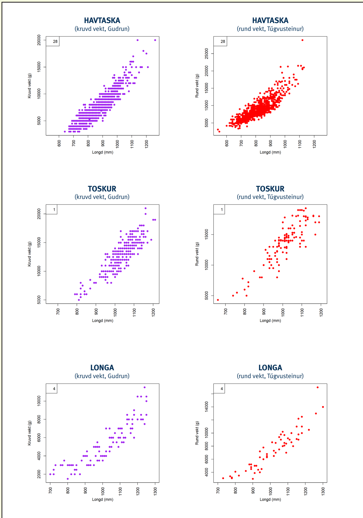
Mynd 2. Longd móti vekt fyri havtasku, tosk og longu frá royndarveiðu á Føroyabanka í 2021. Vektin er krúvd vekt hjá Gudrun og rund vekt hjá Túgvusteini.
