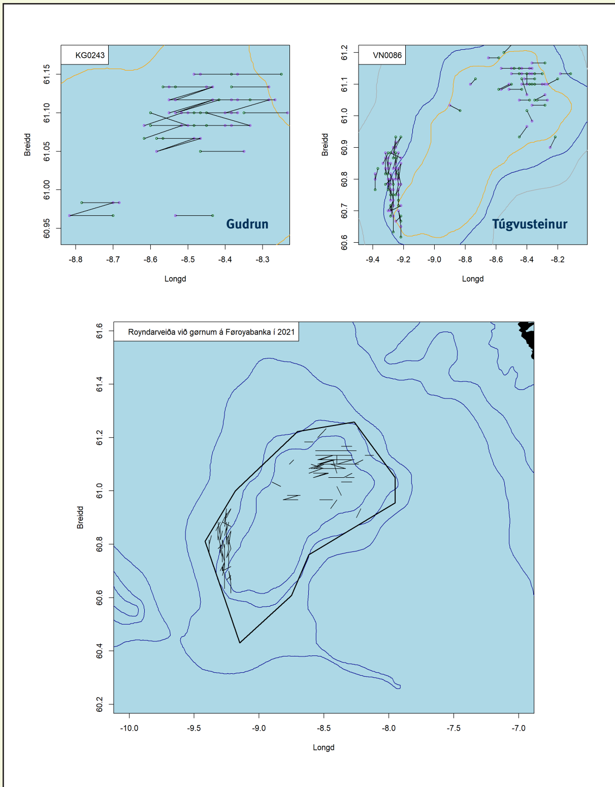
Mynd 1. Garnasetur pr. skip (ovaru myndir) og samlað (niðara mynd) á Føroyabanka í 2021, her teknaðar sum beinar linjur millum byrjanar- og endaposition. Svarta linjan vísir royndarøkið.
