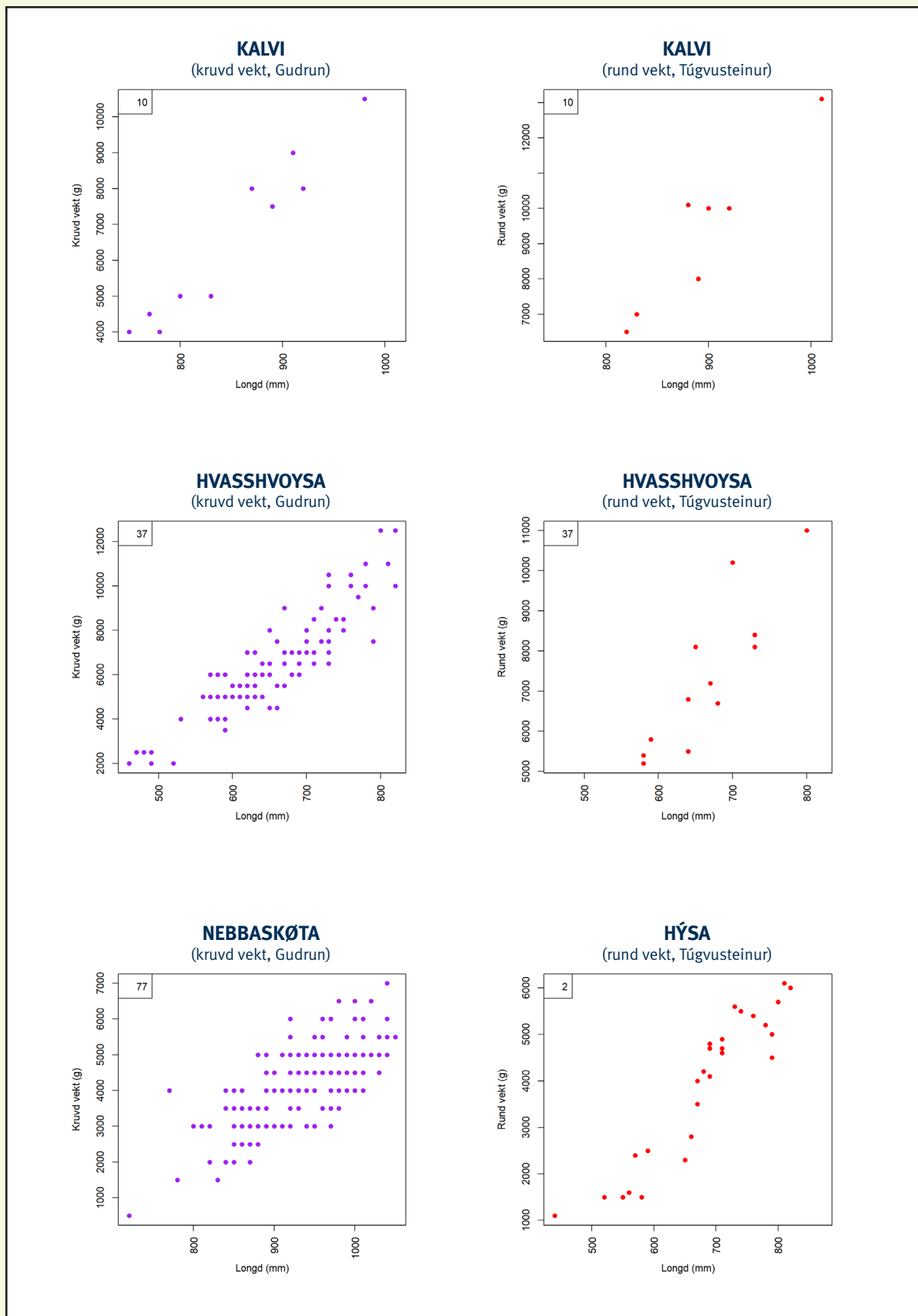
Mynd 3. Longd móti vekt fyri kalva, hvasshvoysu, nebbaskøtu og hýsu frá royndarveidu á Føroyabanka í 2021. Vektin er krudv vekt hjá Gudrun og rund vekt hjá Túgvusteini.
