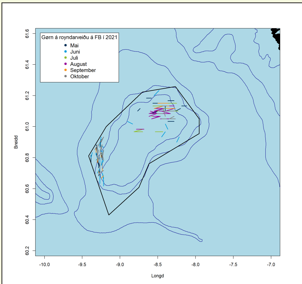
Mynd 5. Gørnasetur littar eftir mána á Føroyabanka í 2021. Svarta linjan vísir royndarøkið.
