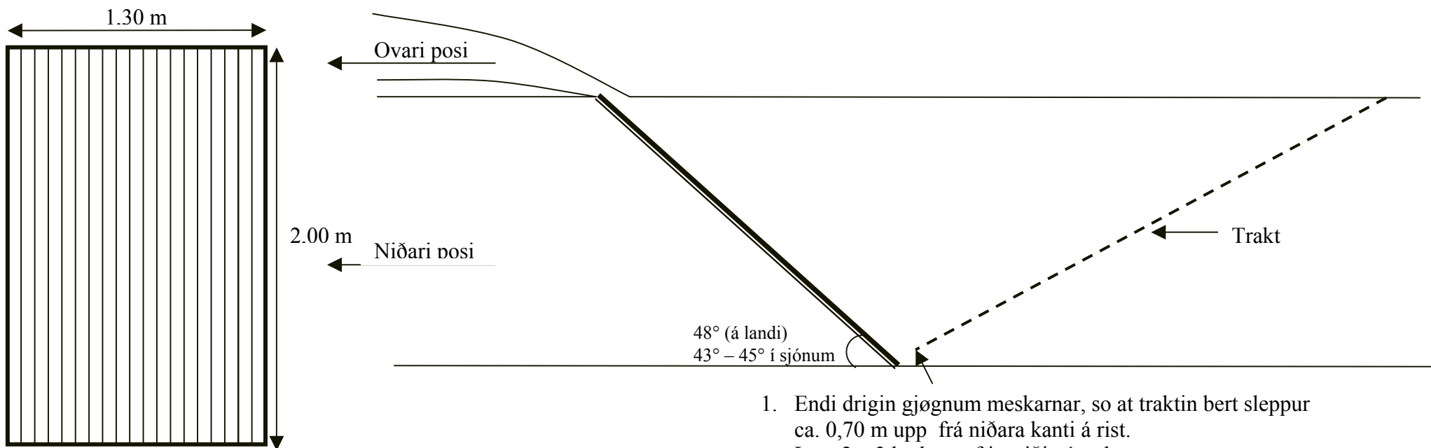
Mynd 3: Rigging av troli og ristum.
