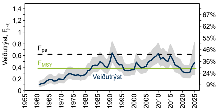
Mynd 4. Veiðutrýst fyri uppsa frá 1961 til 2025, frá stovnsmetingini í 2025. %-virðið høgrumegin vísir, hvussu stórt partur verður fiskaður úr stovninum hvørt ár. Óvissan er víst sum grátt øki. F_{pa} er 0,62 og F_{MSY} er 0,38 (24%).
