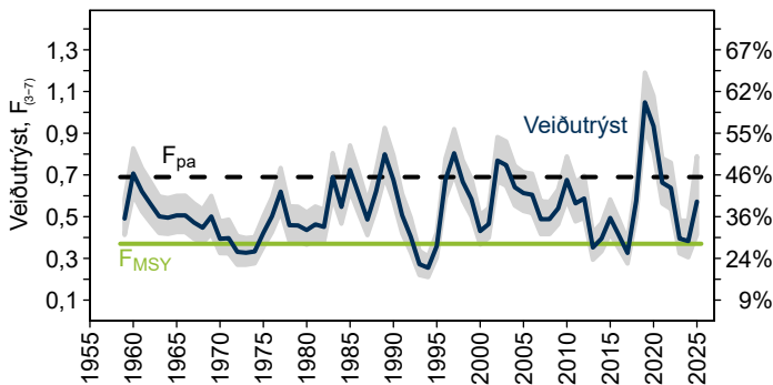
Mynd 12. Veioðutrýst fyri toski á Landgrunninum frá 1959 til 2025, frá stovnsmetingini í 2025. %-virðið høgrumegin vísir, hvussu stórir partur verður fiskaður úr stovninum hvørt ár. Óvissan er víst sum grátt øki. F_{pa} er 0,69 og F_{MSY} er 0,37 (28%).
