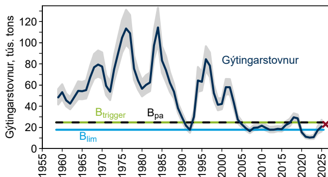
Mynd 3. Gýtingarstovnur av toski á Landgrunninum frá 1959 til 2025, frá stovnsmetingini í 2025. Óvissan er víst sum grátt øki. B_{trigger} og B_{pa} eru 24,7 túsund tons. B_{lim} er 17,8 túsund tons. Reyður krossur forsøgn: 2026=22.933 t.
