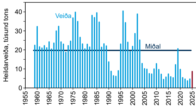
Mynd 9. Heildarveiða av toski á Landgrunninum frá 1959 til 2024. Miðalvirðið er 19,7 túsund tons. Reyður stabbi forsøgn 2025=8.651 t.
