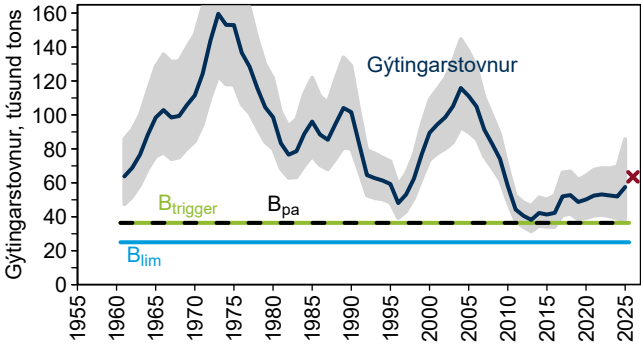
Mynd 1. Gýtingarstovnurin av upsa frá 1961 til 2025, frá stovnsmetingini í 2025. Óvissan er víst sum grátt øki. B_{trigger} og B_{pa} eru 36,4 túsund tons. B_{lim} er 25,0 túsund tons. Reyður krossur forsøgn: 2026=63.521 t.
