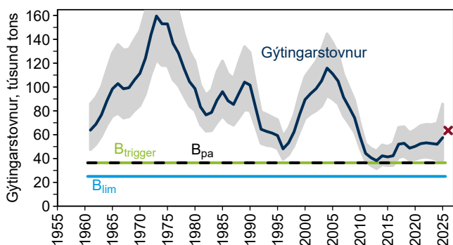
Mynd 3. Gýtingarstovnurin av uppsa frá 1961 til 2025, frá stovnsmetingini í 2025. Óvissan er víst sum grátt øki. B_{trigger} og B_{pa} eru 36,4 túsund tons. B_{lim} er 25,0 túsund tons. Reyður krossur forsøgn: 2026=63.521 t.
