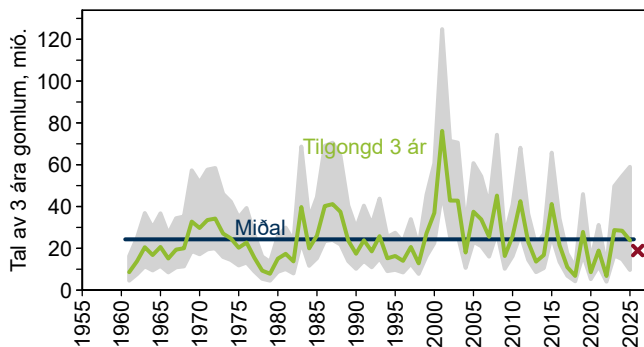
Mynd 2. Tilgongd av 3 ára gomlum uppsa frá 1961 til 2025, frá stovnsmetingini í 2025. Óvissan er víst sum grátt øki. Miðalvirðið er 24,3 milliúnir. Reyður krossur forsøgn: 2026=18.934.
