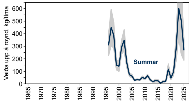
Mynd 14. Veioða upp á roynd av toski frá yvirlitstrolingum hjá rannsóknarskipinum á Føroyabanka á sumri. Veioða upp á roynd er eitt lutfalsligt mál fyri, hvussu stórir stovnurin er. Óvissan er víst sum grátt øki. Miðalvirðið er 296,7 kg/tíma um summarið, árin 1996 til 2002.
