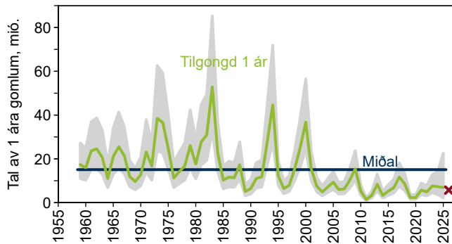
Mynd 10. Tilgongd av 1 ára gomlum toski á Landgrunninum frá 1959 til 2025, frá stovnsmetingini í 2025. Óvissan er víst sum grátt øki. Miðalvirðið er 15,1 milliúnir. Reyður krossur forsøgn: 2026=5.713.
