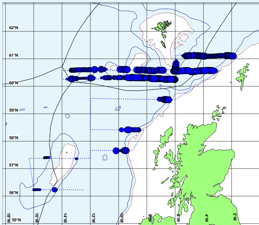
Mynd 1. Akustiskar skrásetingar av svartkjafti ( s_A , m^2/nm^2 ) sunnan fyri Føroyar 23/3-6/4 2022. Nøgðin er víst sum sirklar, har støddin á sirklinum vísir, hvussu nógv av svartkjafti stóð undir skipinum. 200 og 500 botnlinjur eru vístar.
