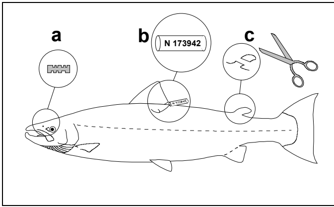
Figur 3.2.1. Ulike merkemeter for laks a) innvendig mikromerke, b) utvendig merke og c) fettfinne klipping (brukes alltid ved innvendig merking).
