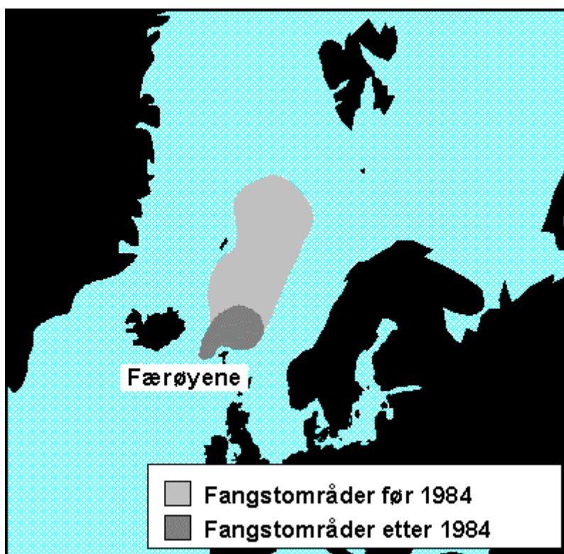
Figur 2.1.1. Kart over Færøyske fangstområder i Norskehavet siden slutten av 70-årene. Fangstområder før og etter NASCO (North Atlantic Salmon Conservation Organisation) ble opprettet i 1984 er indikert.
