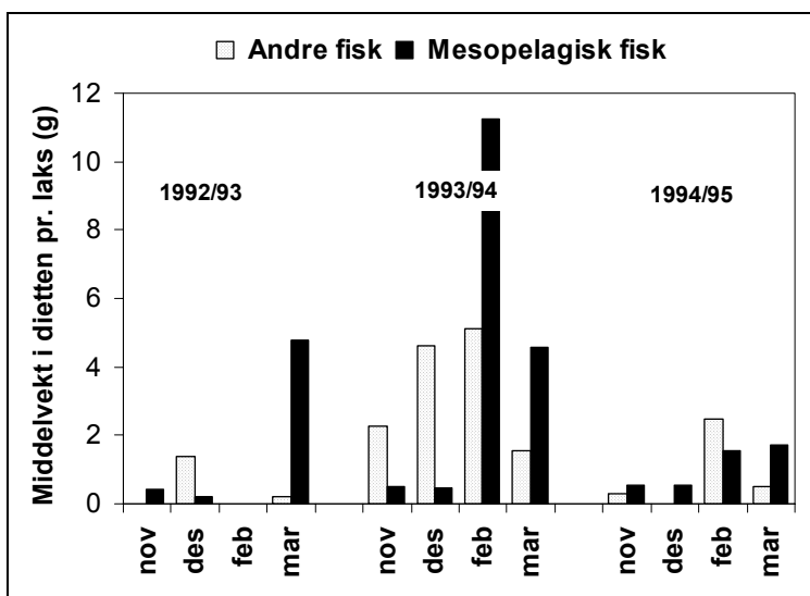
Figur 4.5.5. Sammenligning av mesopelagiske fisk (Lakssild, lysprykkfisk og laksetobis) og andre fisk i dietten (middelvekt i g pr. laks) pr. måned i tre fangstsesonger 1992/93-1994/95.
