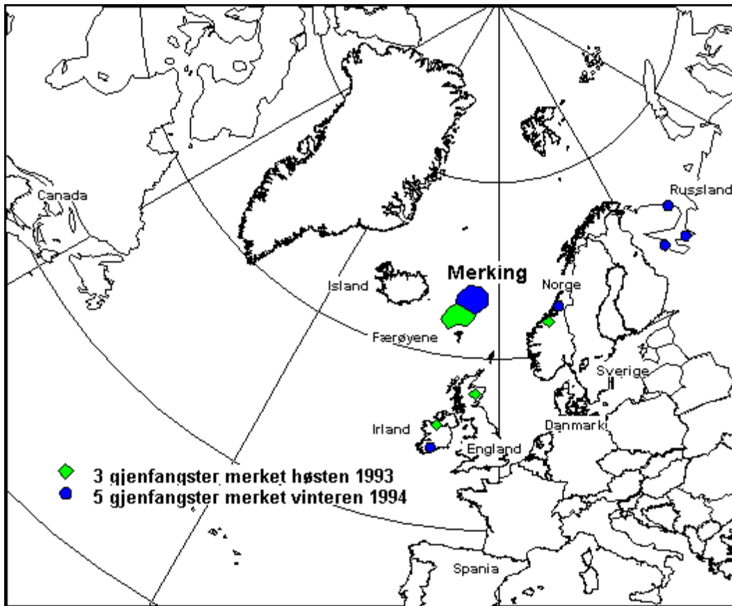
Figur 4.2.5. Gjenfangst av villaks merket i 1993/94 sesongen ved Færøyene.
