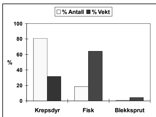
Figur 4.5.1. Fordeling av mageinnhold i antall (%N) og vekt (%W) av hovedgruppen av byttedyr for laks i tre fiskesesonger 1992/93-1994/95 nord for Færøyene.
