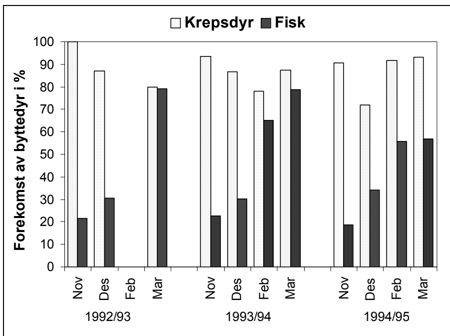
Figur 4.5.4. Forekomst i prosent (%F) av bytte av typen krepsdyr (crustacea) i forhold til fisk pr. måned i laksemagene gjennom tre fiskesesonger 1992/93-1994/95 fra området nord for Færøyene.
