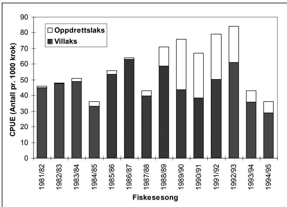
Figur 4.4.3. CPUE (fangst i antall pr. 1000 krok pr. dag) av villaks (mørk søyle) og rømt oppdrettslaks (lys søyle) i fisket ved Færøyene siden 1981/82 sesongen. Forskningsfiske med kun en båt har vært i drift siden 1991/92 sesongen.
