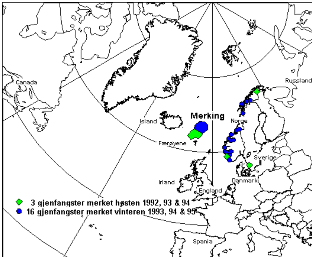
Figur 4.2.7. Geografisk fordeling av gjenfangster av rømt oppdrettslaks merket ved Færøyene høst (nov-des) og vinter (feb-mar) i perioden 1992-95.
