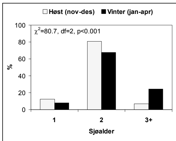
Figur 4.3.2. Sjøalder fordeling av villaks ved Færøyene i perioden 1991/92-1994/95.
