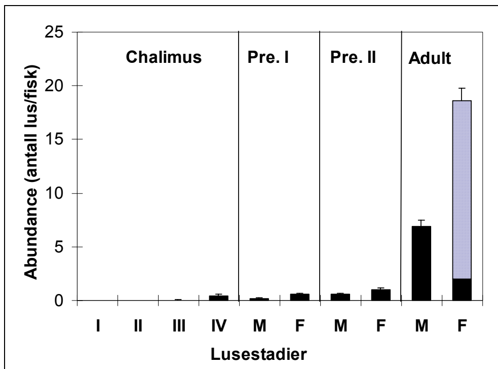
Figur 4.6.2. Abundans (+ standard feil) av Lepeophtheirus salmonis på 127 laks i Norskehavet, fra mars 1993 (3 laks), februar-mars 1994 (13 laks) og fra november 1994 til mars 1995 (111 laks). Notasjon: Pre.=preadult, M=hann og F=hunn. Skravert søyle (lysere) representerer andel gravide hunner.
