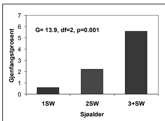
Figur 4.2.2. Gjenfangstprosent fordelt på sjølager. Antall gjenfangster av 1, 2 og 3 sjøvinter laks var henholdsvis 2, 71 og 14 individer.
