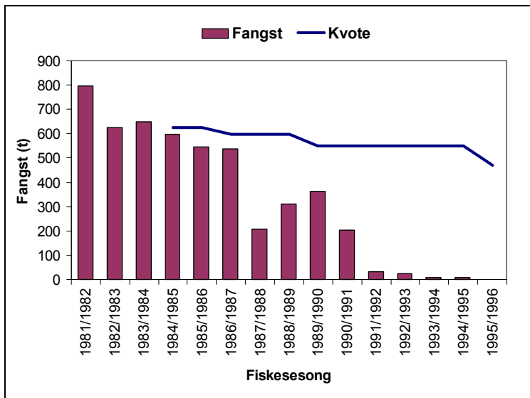
Figur 2.1.4. Fangst av Atlantisk laks ved Færøyene fra 1981/82 sesongen til i dag. Laksekvote tildelt av NASCO (North Atlantic Salmon Conservation Organisation) er indikert som strek over fangsttallene. Siden 1991 har kun én forskningsbåt fisket da kvoten har vært kjøpt opp.
