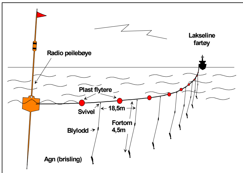
Figur 2.1.3. Figur av lakseline brukt i Norskehavet av Færøyske laksefiskere.
