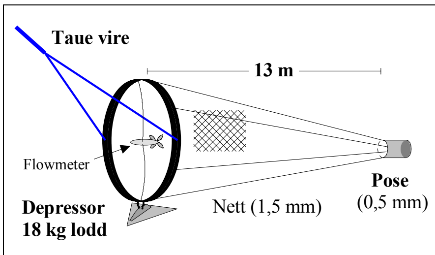
Figur 3.5.2. Plankton nett (MIK) til innsamling av byttedyr i områdene hvor laksefisket foregikk.
