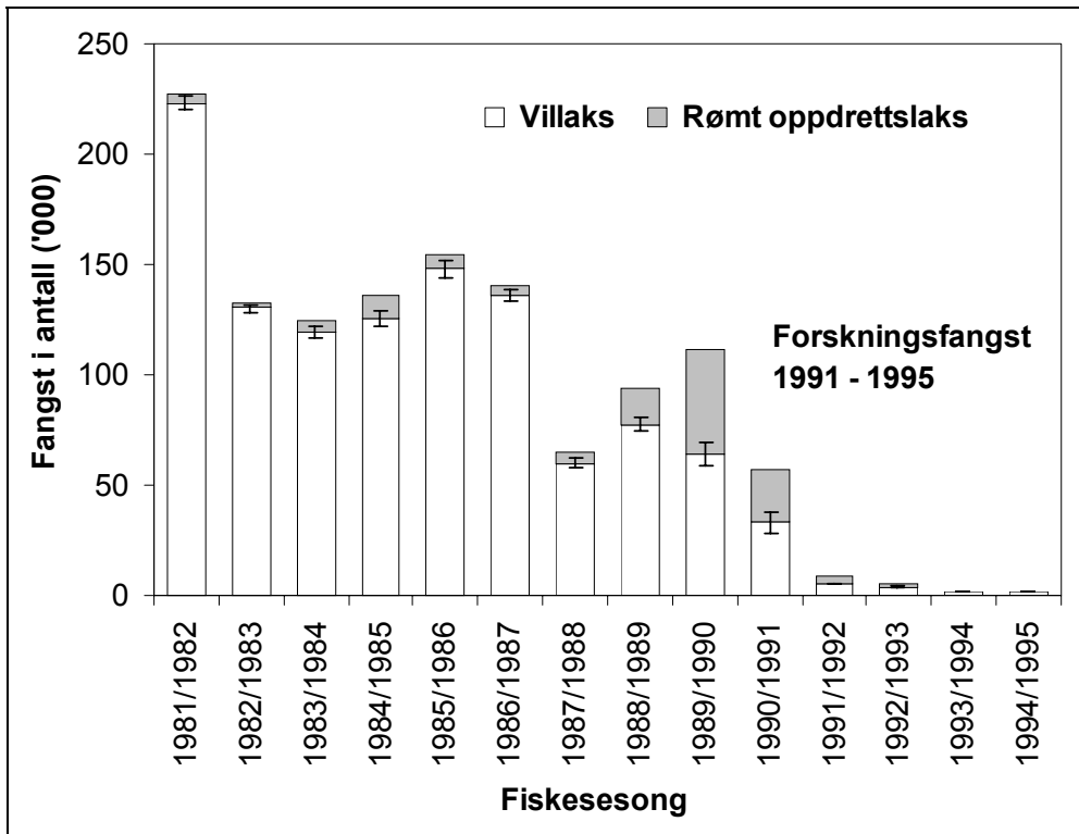
Figur 4.4.2. Fangst av vill (åpen søyle) og oppdrettet laks (skravert søyle) nord for Færøyene og i Norskehavet siden 1981/82 sesongen. Konfidensintervaller (95%) er vist i overgangen mellom villaks og rømt oppdrettslaks hvert år. De lave fangstene fra 1991 til 1995 skyldes at det ikke har vært kommersielt fiske og at kun en forskningsbåt har vært i drift i området.
