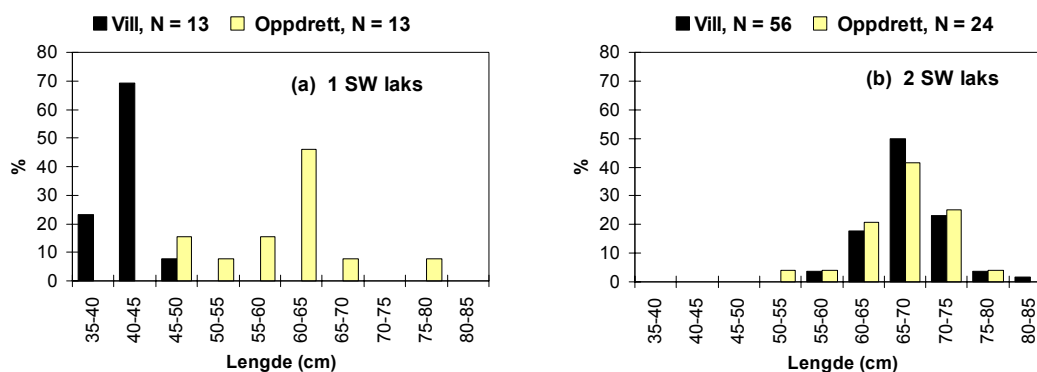
Figur 4.6.1. Lengdefordeling av villaks og rømt oppdrettslaks undersøkt for lakselus i 1994/95 sesongen, (a) 1SW (1 sjøvinter) laks og (b) er 2SW laks.
