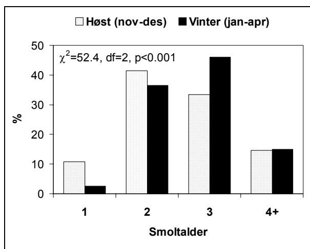
Figur 4.3.1. Smoltalder fordeling av villaks ved Færøylene 1991/92-1994/95.
