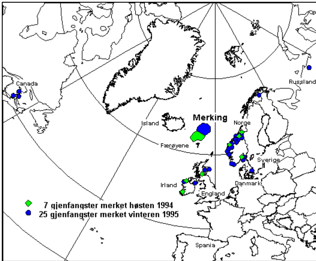
Figur 4.2.6. Gjenfangst av villaks merket i 1994/95 sesongen ved Færøyene.
