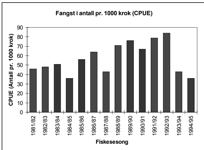
Figur 2.1.5. Fangst pr. redskapsenhet (antall fisk pr. 1000 krok pr. dag) i Færøyfisket siden 1981/82 sesongen. Siden 1991 har kun én forskningsbåt fisket da kvoten har vært kjøpt opp.
