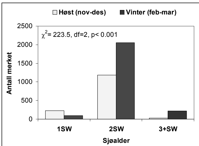
Figur 3.2.3. Sjælalder av villaks som ble merket og satt ut igjen om høsten og vinteren i Norskehavet.
