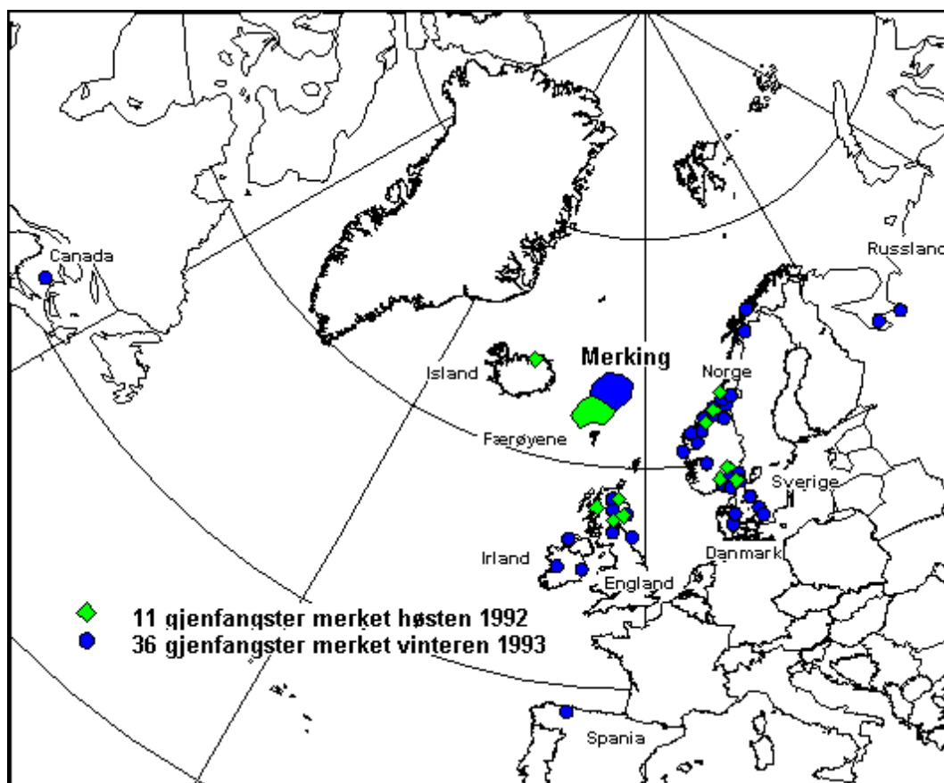
Figur 4.2.4. Gjenfangst av vill laks merket i 1992/93 sesongen ved Færøyene.
