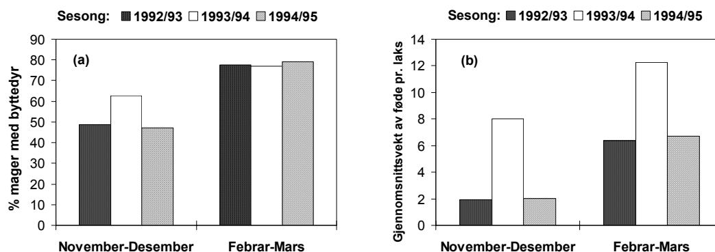
Figur 4.5.3. (a) Andel av laks med mager som inneholder bytte (ikke tomme mager) fordelt på høst (nov-des) og vinter (feb-mar) i tre fiskesesonger 1992/93-1994/95, og (b) gjennomsnittsvekt av byttedyr (g) pr. laks om høsten og vinteren samme periode.
