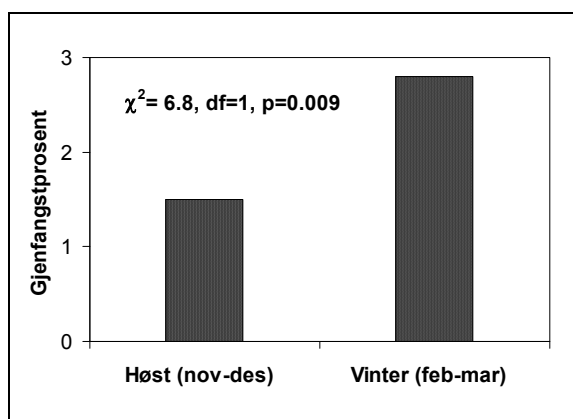
Figur 4.2.3. Gjenfangstprosent av laks merket ved Færøyene om høsten (nov-des) og om vinteren (feb-mar) fra 1992-1995. Villaks og rømt oppdrettslaks er slått sammen.
