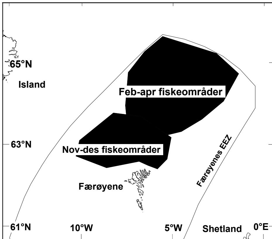
Figur 3.1.1. Kart over fangstområder for laks i Norskehavet under forskningsprogrammet ved Færøyene (1992-95). Fisket finner sted relativt nær land om høsten og forflyttes i nordøstlig retning om vinteren.
