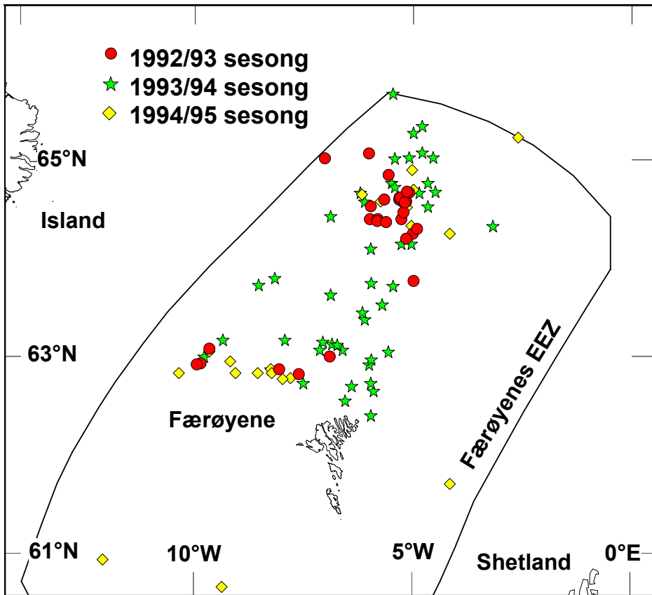
Figur 3.5.1. Kart over fangstposisjoner hvor mageprøver ble samlet inn i 1992/93, 1993/94 og 1994/95 sesongene nord for Færøyene.
