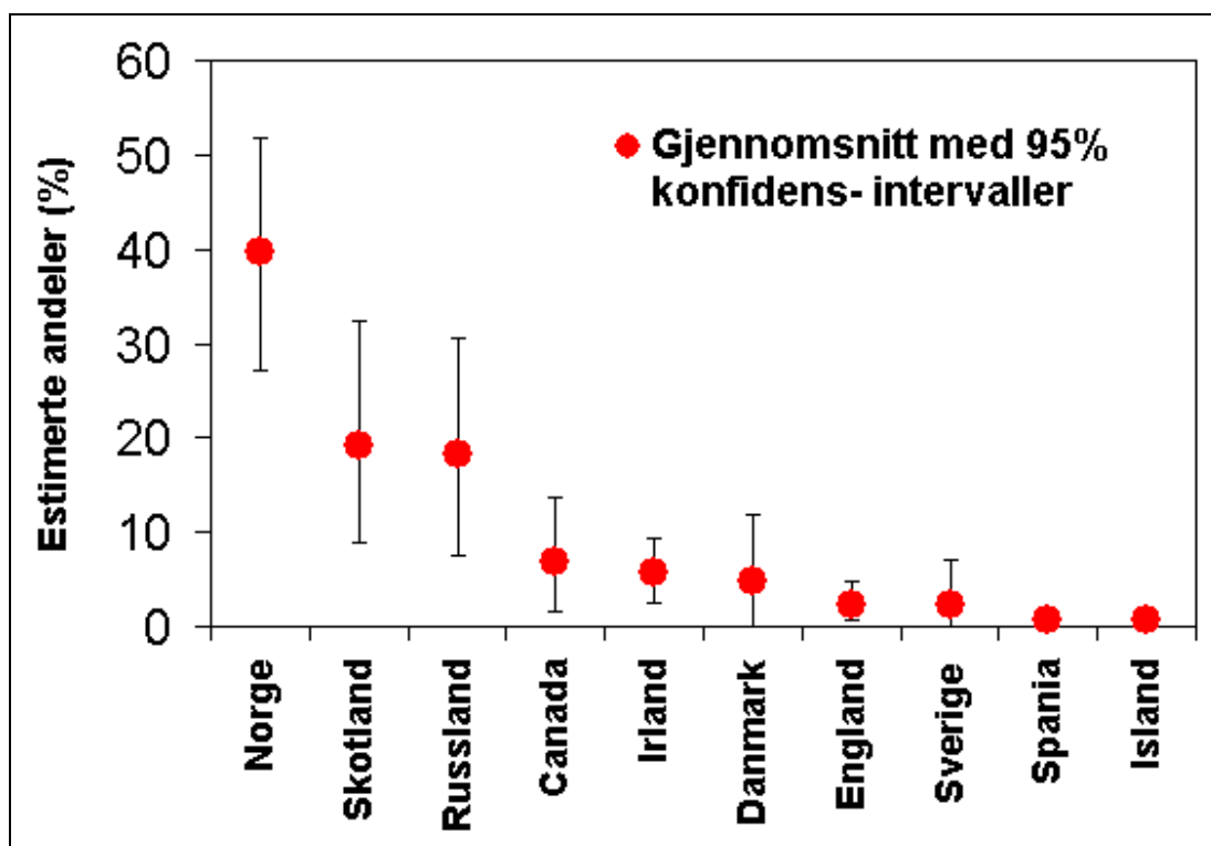
Figur 4.2.8. Estimerte prosentandeler (med 95% konfidensintervaller) av laks gjenfanget i respektive opprinnelsesland, som ble merket og satt ut ved Færøyene i perioden 1992-1995.
