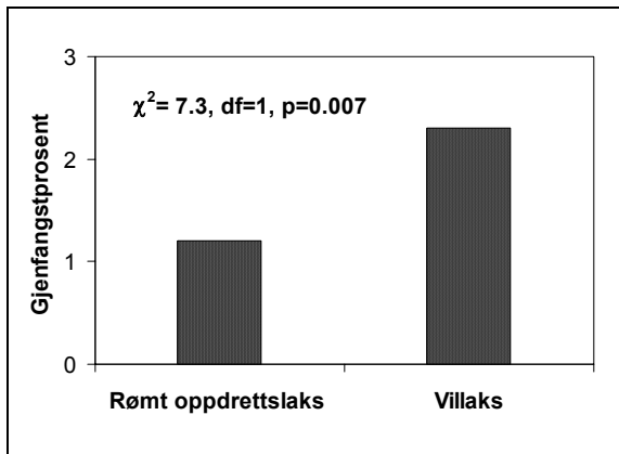
Figur 4.2.1. Gjennomsnittlig gjenfangstprosent av villaks og rømt oppdrettslaks merket ved Færøyene 1992-1995.
