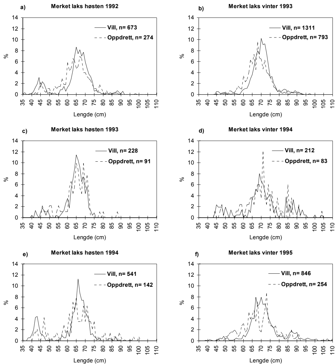
Figur 3.2.2. Lengdefordeling av villaks og rømt oppdrettslaks som ble merket og satt ut igjen om høsten og vinteren i Norskehavet.
