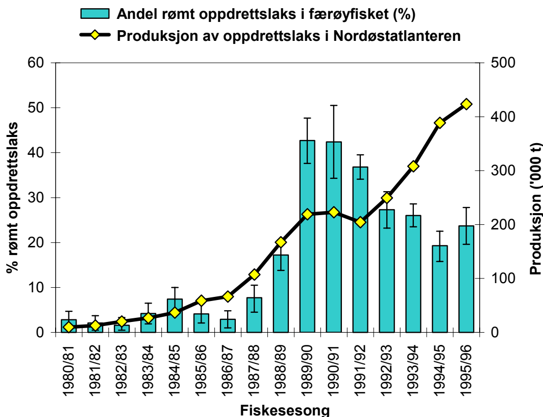
Figur 4.4.1. Tidsserie av andel rømt oppdrettslaks i prøver tatt ved Færøyene siden 1980 og produksjon av oppdrettslaks i det nordøstlige Atlanterhavet.
