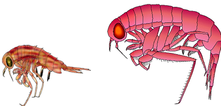
Figur 4.5.2. Tegning av Themisto compressa f. compressa og T. libellula , to av de hyppigst forekommende byttedyr i laksemagene.
