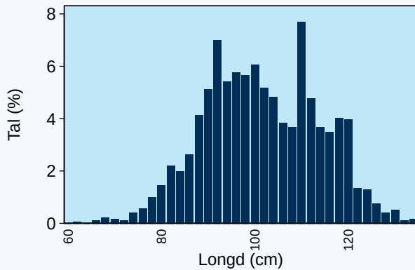
Mynd 8. Longdarbýtið í blálonguveiðuni undir Føroyum í 2019. Longdirnar eru bólkaðar fyri hvørjar 2 cm, t.v.s. at bólkurin 70 cm eru blálongur, sum eru 70 og 71 cm.
