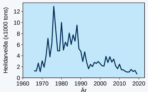
Mynd 7. Heildarveiðan av blálongu undir Føroyum 1966-2019 í rundari vekt.
