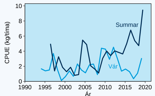
Mynd 10. Veiða upp á roynd av blálongu hjá Magnusi Heinasyni á yvirlitstrolingunum á Landgrunninum um várið (1994-2019) og um summarið (1996-2019).
