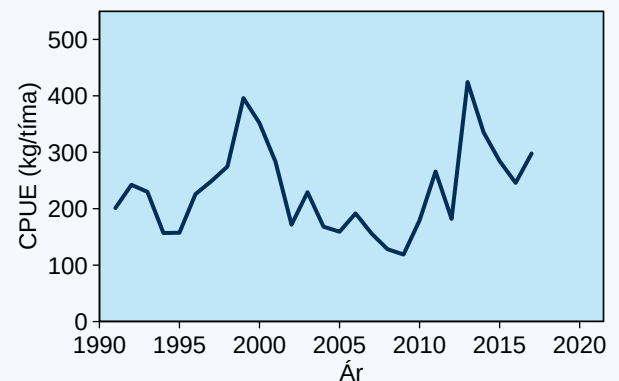
Mynd 9. Veiða upp á roynd av blálongu hjá trolarum undir Føroyum (1991-2017).
