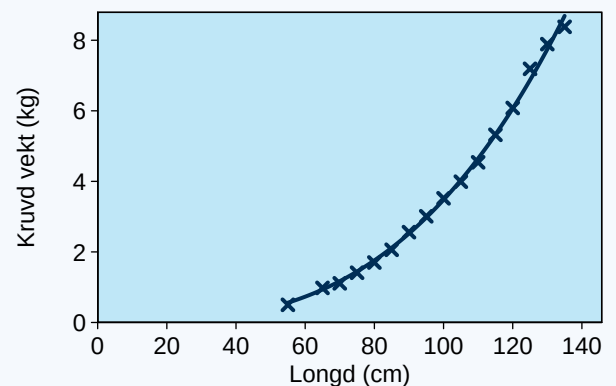
Mynd 4. Longd móti vekt mátað frá landingum, árin 2015-2019.
