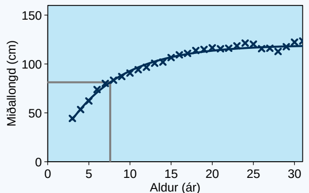
Mynd 2. Miðallongd móti aldri mátað á ymiskum túrum við Føroyar 1987-1999. Víst er, nær helvtin av blálongunum er búgvinn at gýta fyrstu ferð.
