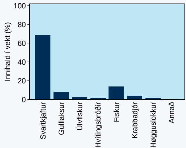
Mynd 6. Føðin í vekt í blálongumagum býtt í høvuðsbólkar árin 2014-2019.
